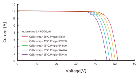
電流 - 電圧曲線
