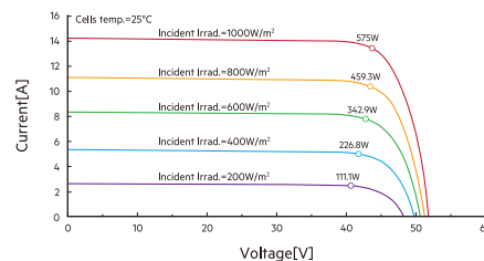
電流 - 電圧曲線
