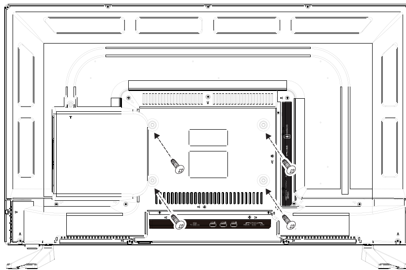
取り付けネジM6×10×4本
